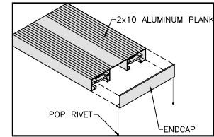
End Cap
